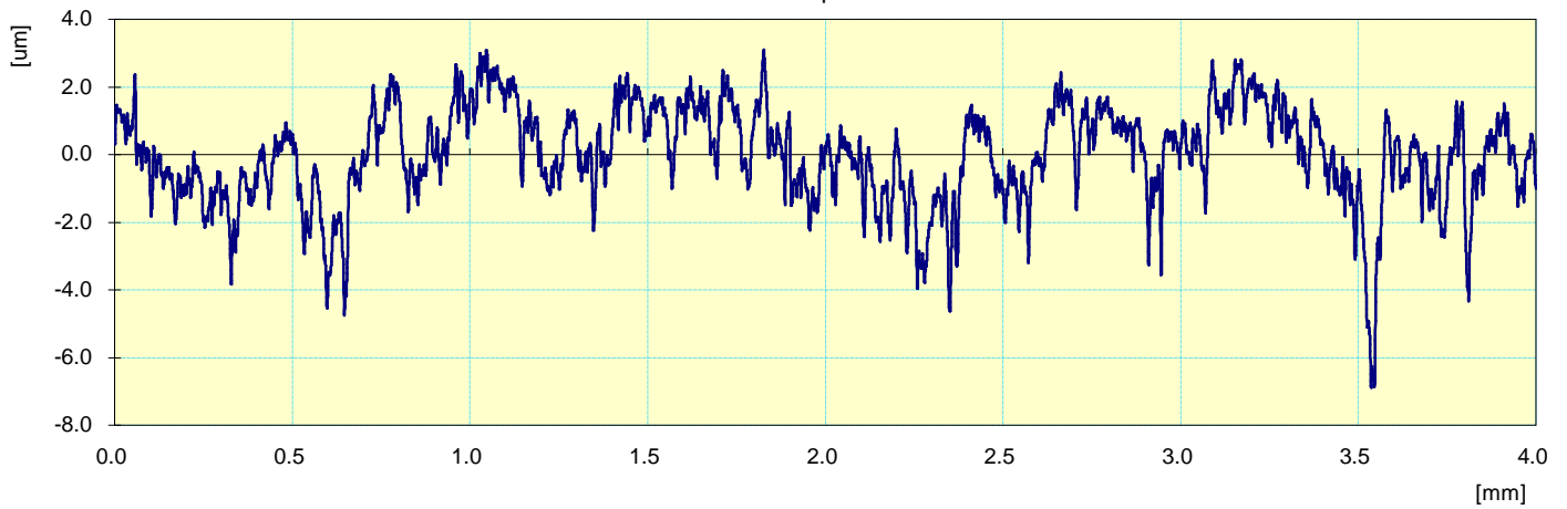
Gemeten profiel
