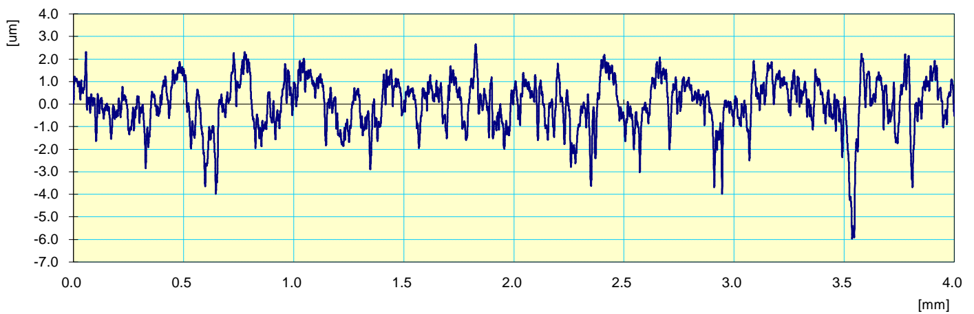
RProfiel
